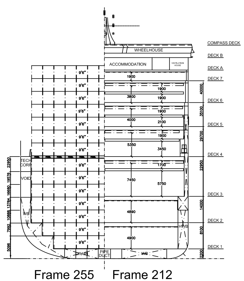
Frame 255 Frame 212
